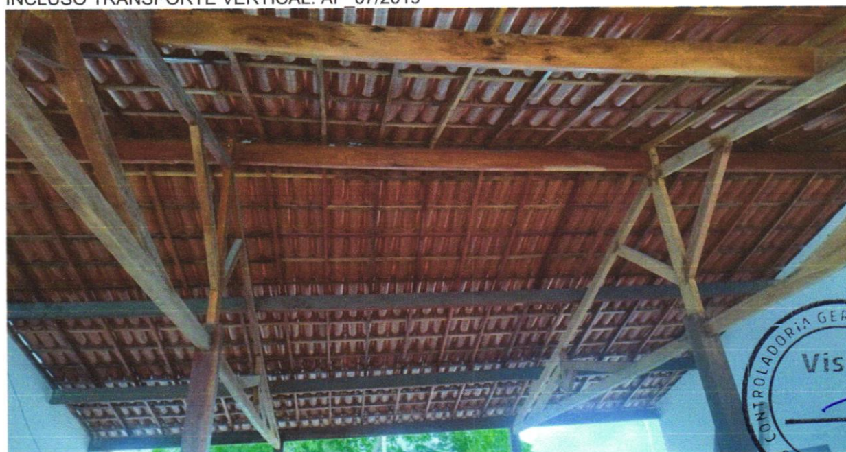
FOTO 20 - TRAMA DE MADEIRA COMPOSTA POR TERÇAS PARA TELHADOS DE ATÉ 2 ÁGUAS PARA TELHA ONDULADA DE FIBROCIMENTO, METÁLICA, PLÁSTICA OU TERMOACÚSTICA, INCLUSO TRANSPORTE VERTICAL. AF_07/2019
