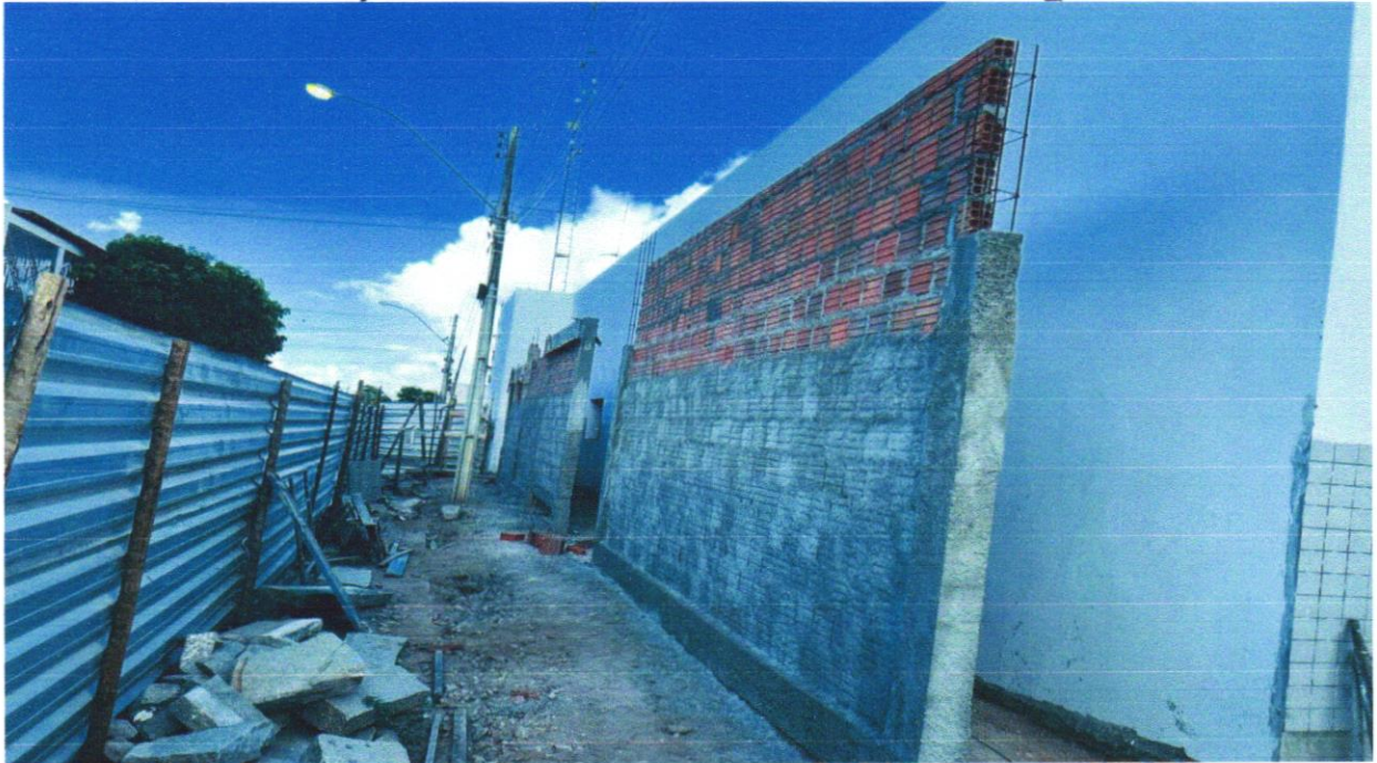
FOTO 21 (COMPOSIÇÃO REPRESENTATIVA) EXECUÇÃO DE ESTRUTURAS DE CONCRETO ARMADO, PARA EDIFICAÇÃO INSTITUCIONAL TÉRREA, FCK = 25 MPA. AF_01/2017
